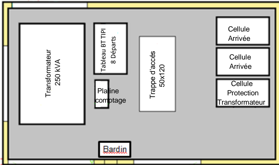
DISPOSITION EQUIPEMENTS
