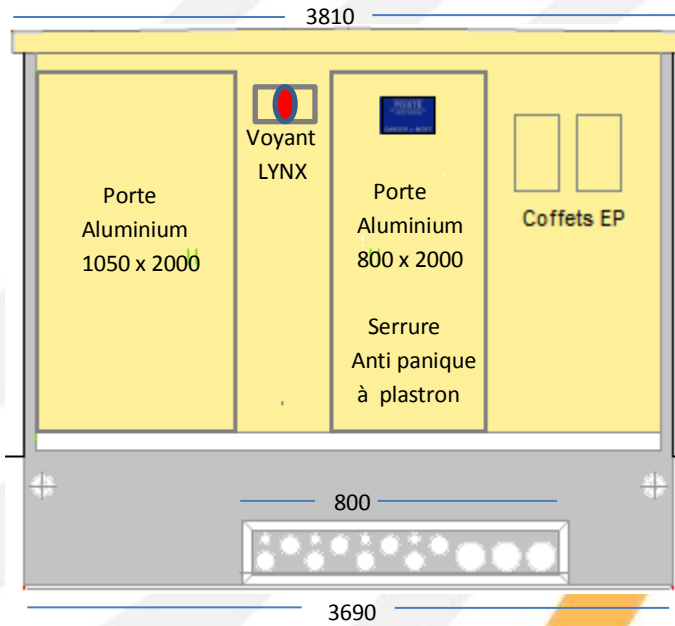
FAÇADE DROITE
